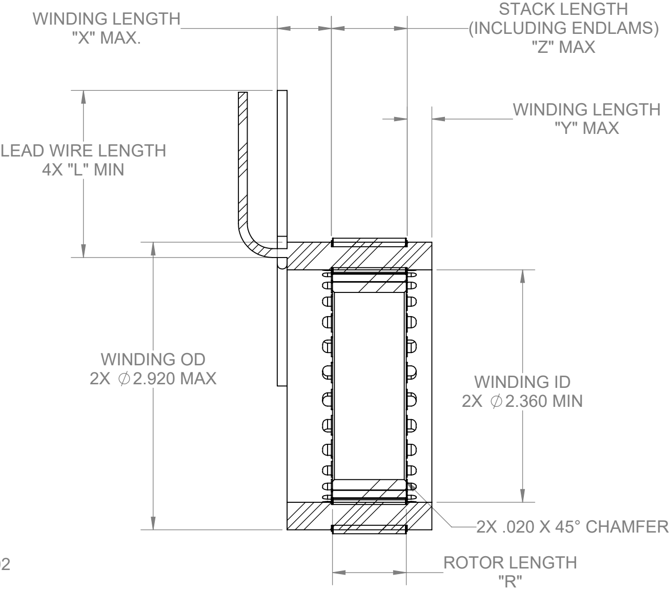
SECTION A-A
